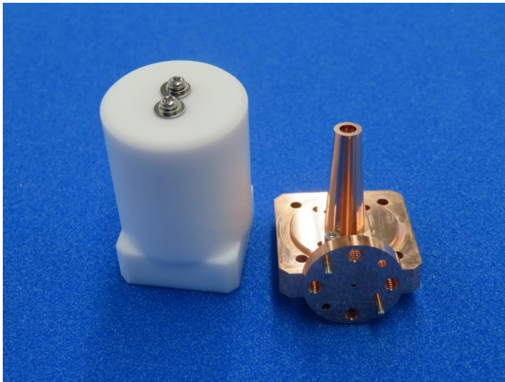
300GHz オムニアンテナ
